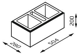
BH28 stĺpcový/múrikový blok
