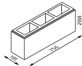
RM19 stĺpcový/múrikový prístrešok
