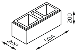
BH20, RP20, RD20 stĺpcový/múrikový blok
