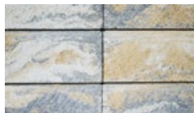
milos
