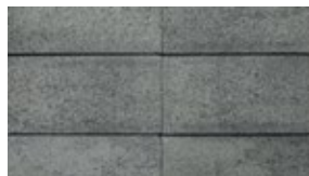
gagat
