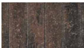
bronzit
