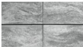
galena
